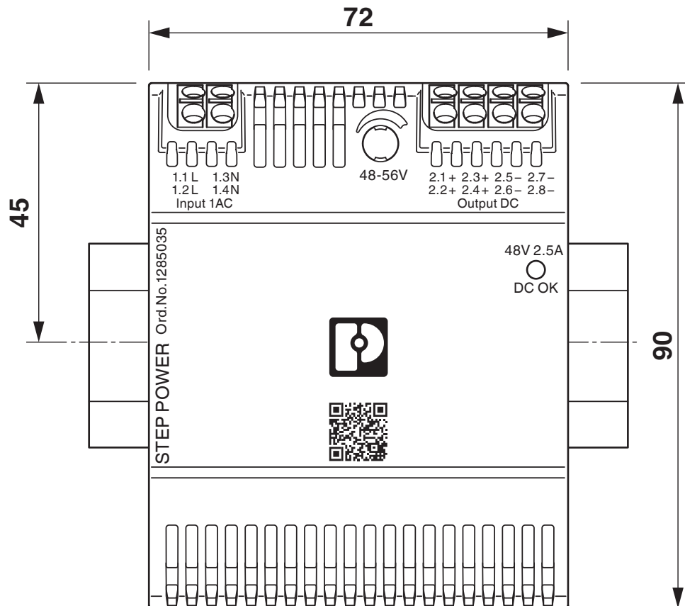
Maßzeichnung
