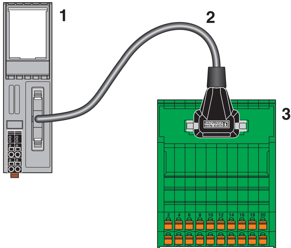
Conexión de un módulo de transferencia
