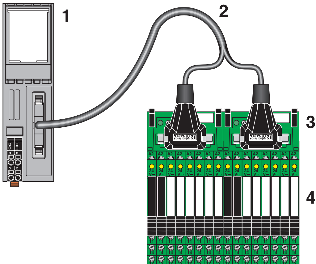
Conexión de módulos de relé
