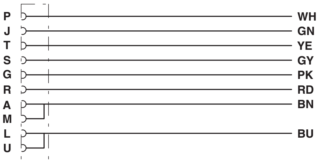
Diagrama eléctrico
