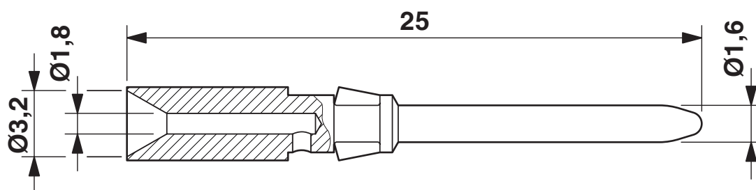
Maßzeichnung
