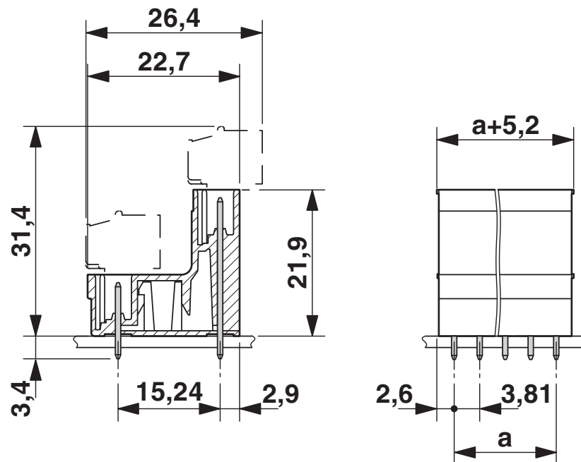
Maßzeichnung
