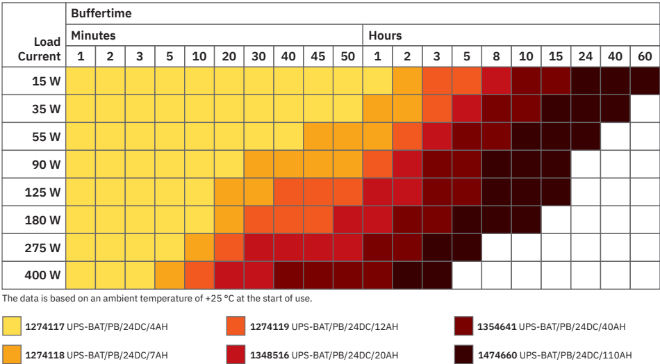
Durées d'autonomie QUINT AC UPS 500 VA pour module de batterie PB
