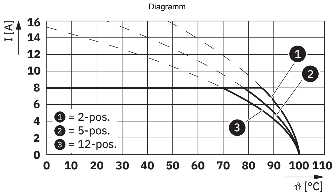
Typ: FK-MCP 1,5/...-STF-3,5 mit MC 1,5/...-GF-3,5 P... THR
