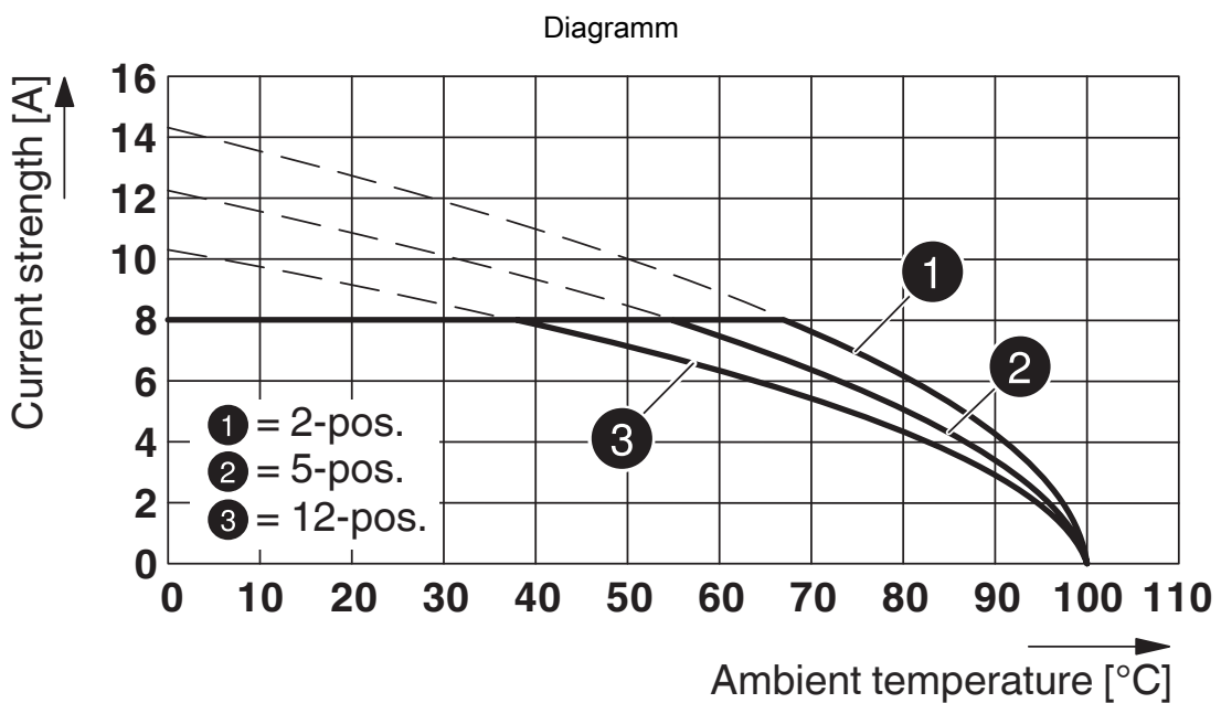
Typ: MCV(W/R) 2,5/...-STF-3,5 mit MC 1,5/...-GF-3,5 P...THR
