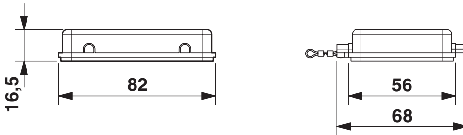
Maßzeichnung
