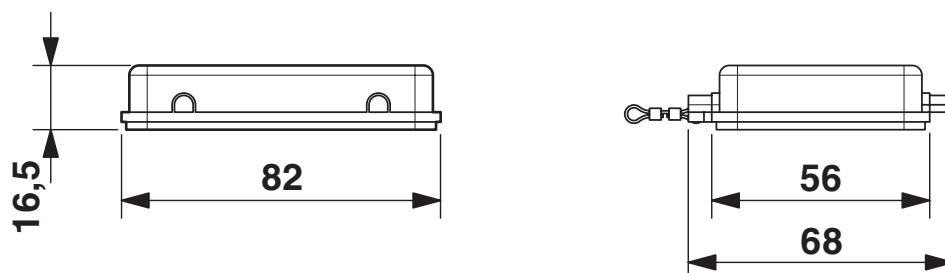
Dessin coté
