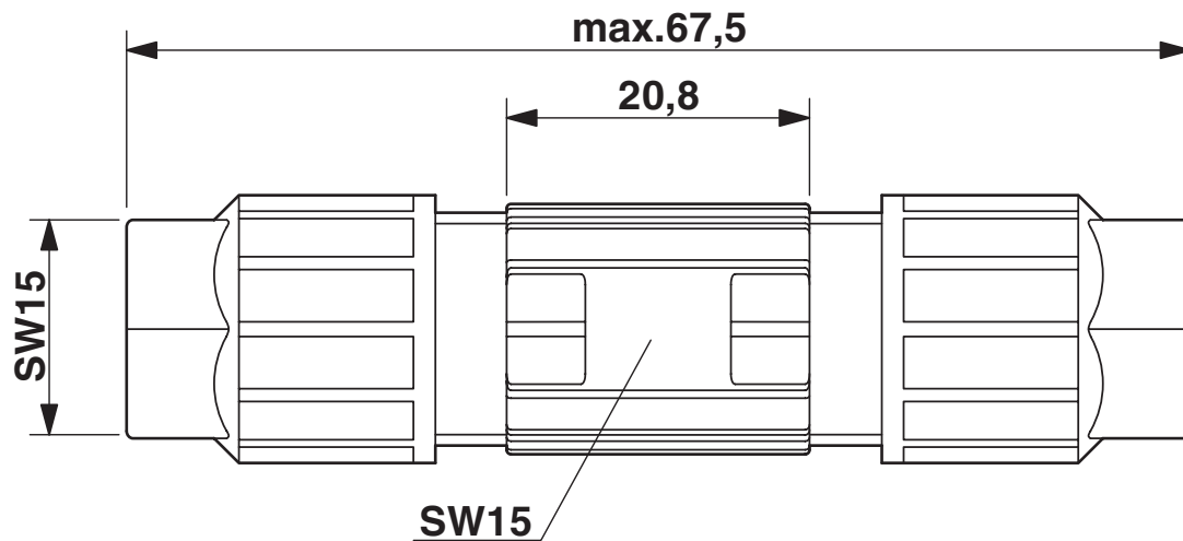
Maßzeichnung
