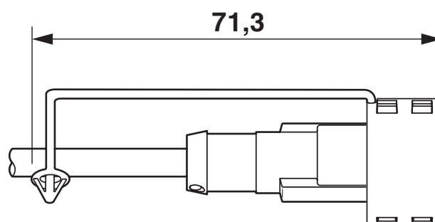
Esquema de dimensiones
