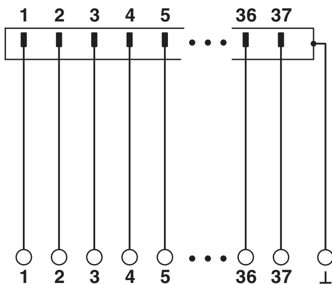
Diagrama eléctrico
