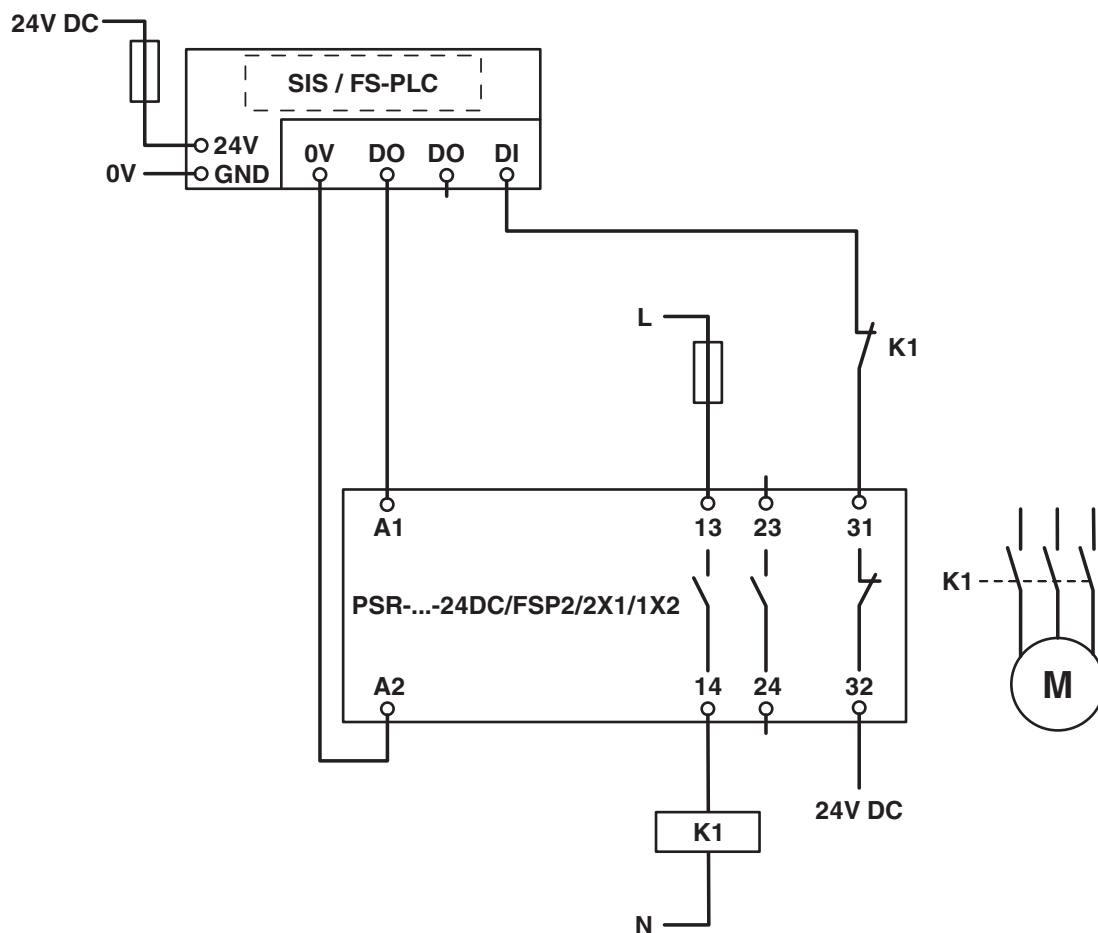
Einkanaliger Anschluss mit Einbindung des Rückmeldestrompfades
