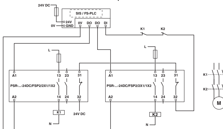
Zweikanaliger Anschluss mit Einbindung des Rückmeldestrompfades
