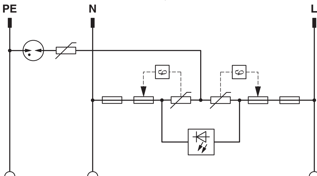
Schaltplan
