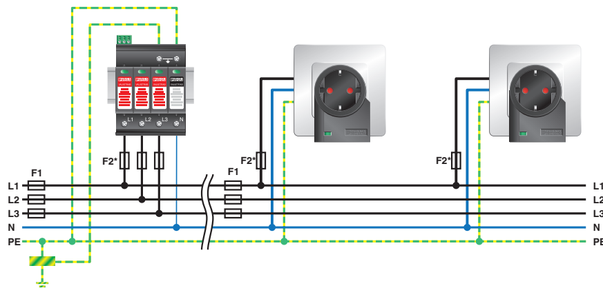
Applikationszeichnung
