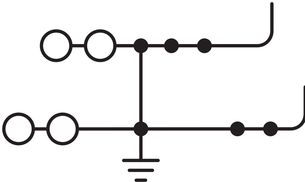
Schaltplan
