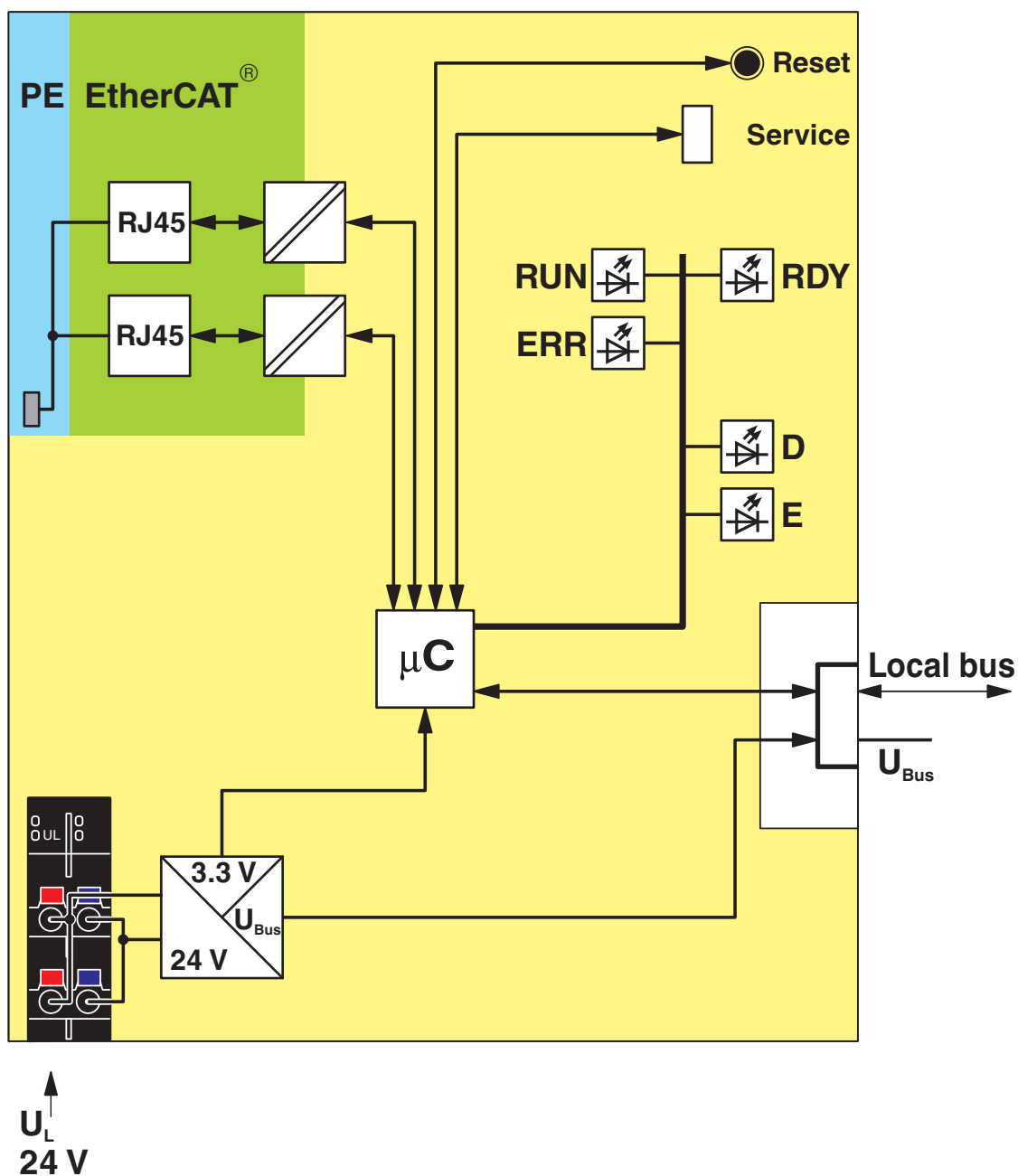
Schéma fonctionnel
