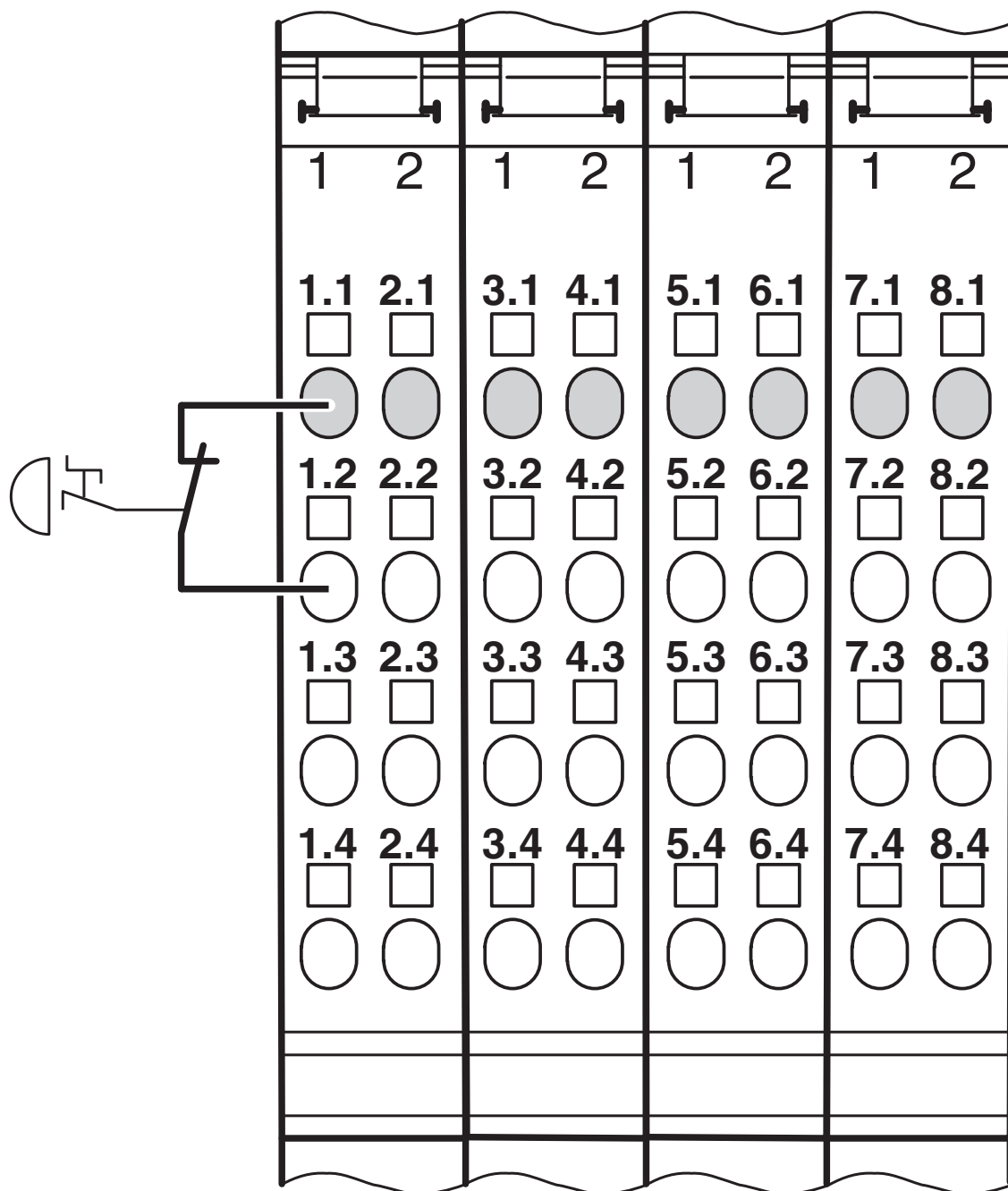
Conexión típica de un circuito de parada de emergencia
