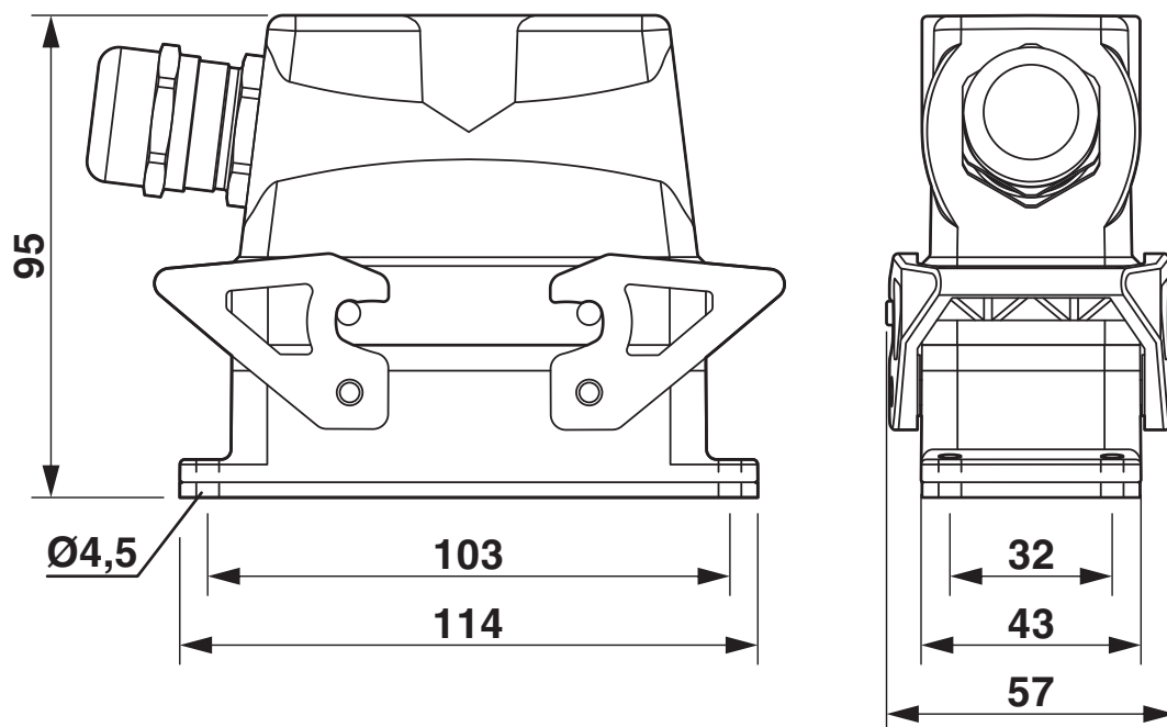
Dessin coté
