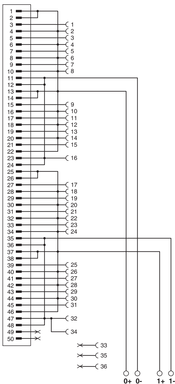
Diagrama eléctrico
