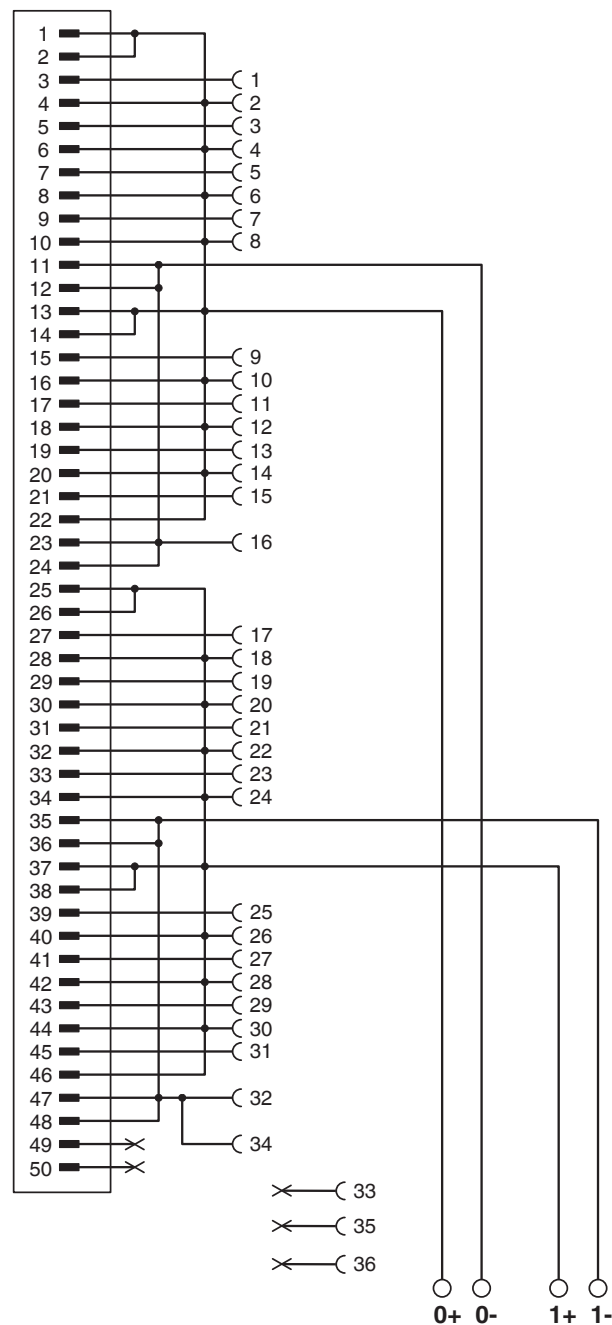
Schéma de connexion
