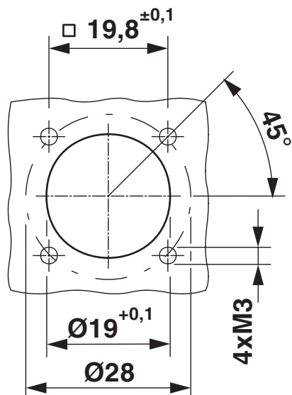
Plano esquemático
