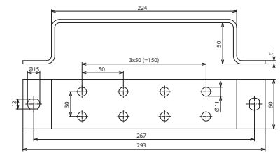
Maßbild ES 2X4 ASB11 V2A
