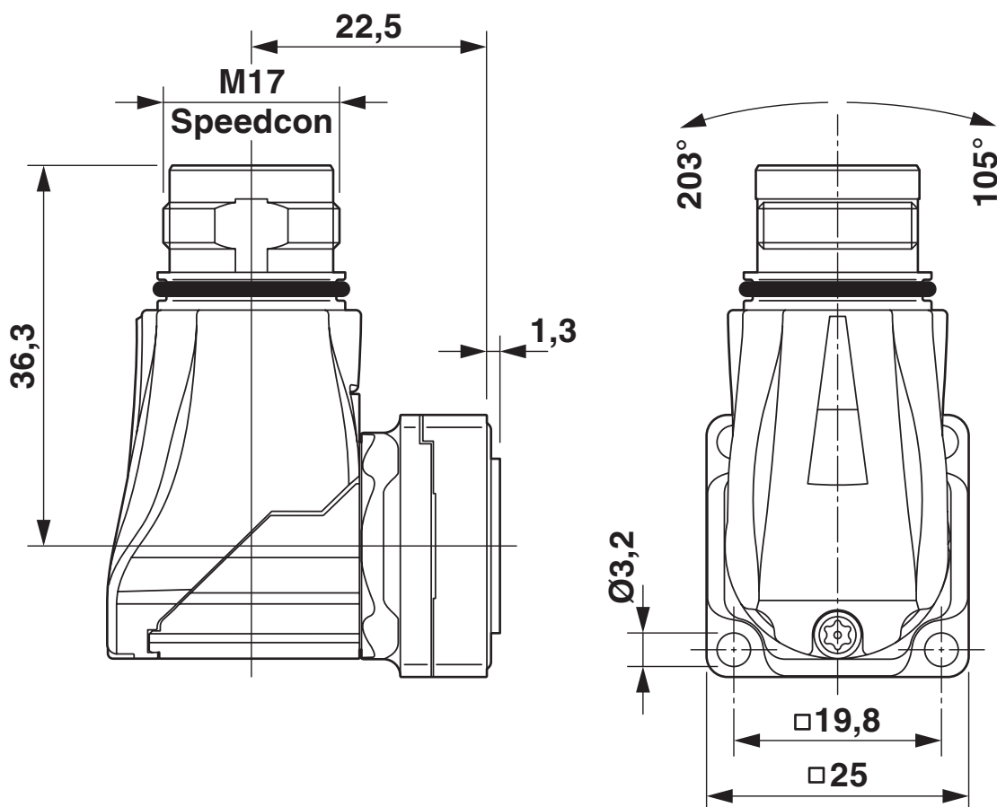
Dessin coté
