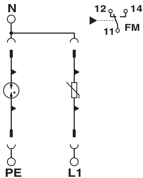
Schaltplan
