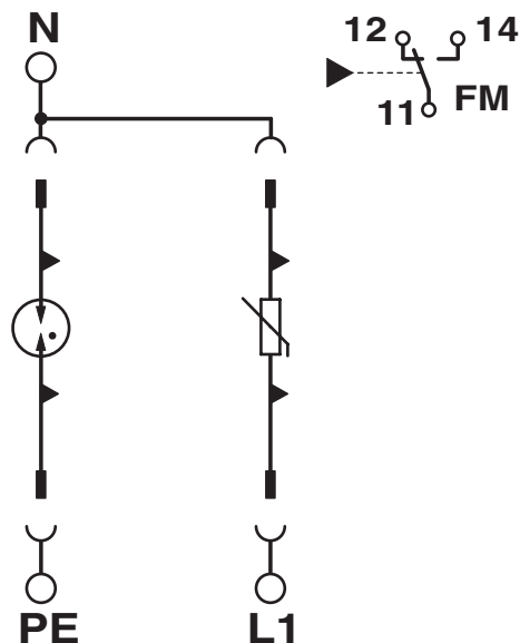
Diagrama eléctrico
