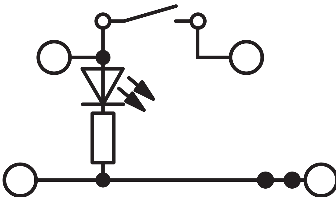
Diagrama eléctrico
