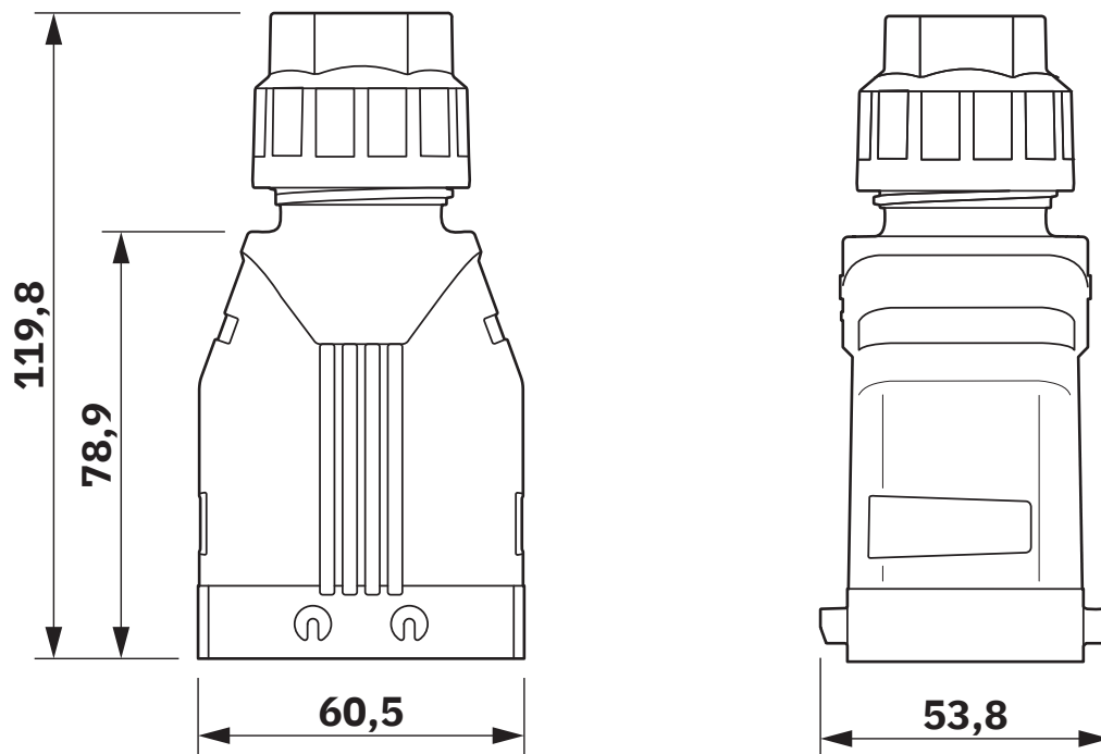
Maßzeichnung
