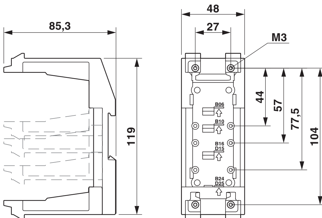
Dessin coté
