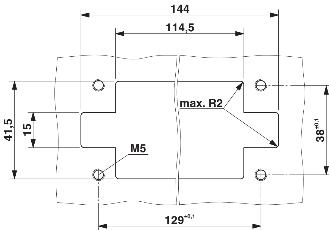
Maßzeichnung
