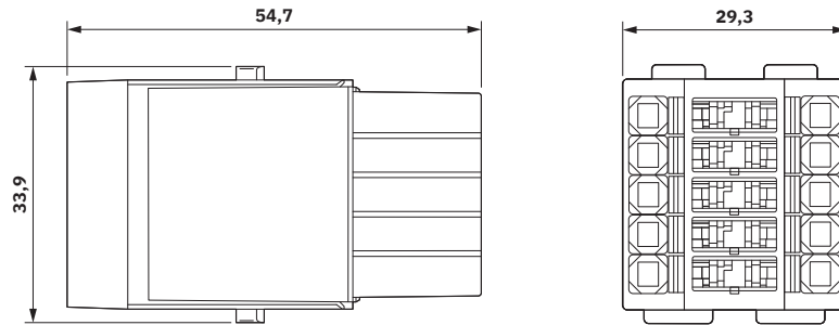
Maßzeichnung
