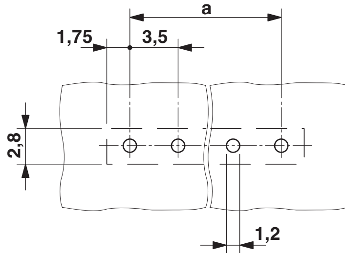
Bohrplan/Lötpadgeometrie
