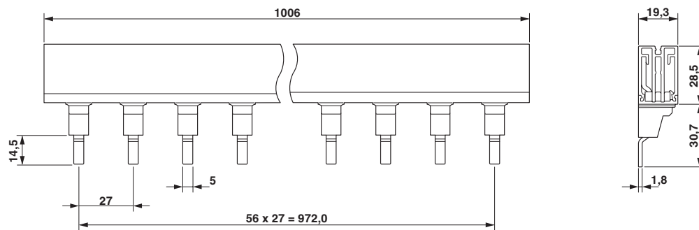
Maßzeichnung
