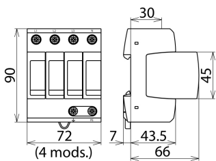
Dimensiones del DG M TNS 275
