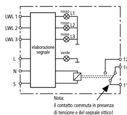
Schema di principio DSI E 3
