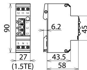
Dimensioni DSI E 3
