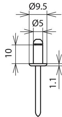
Maßbild BN 5X10 AL V2A
