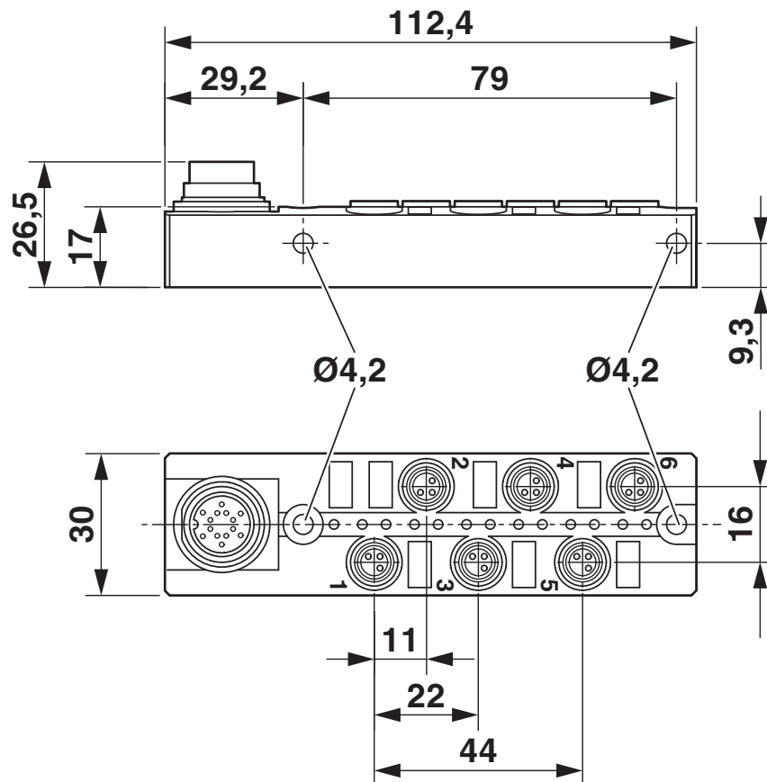
Maßzeichnung
