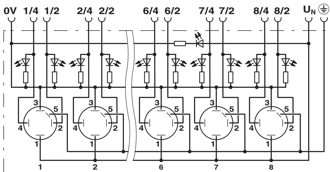
Diagrama eléctrico
