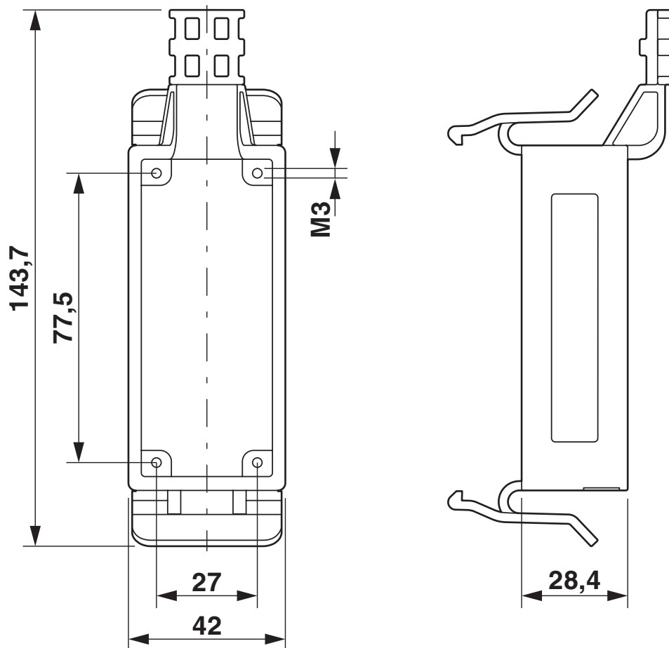
Dessin coté
