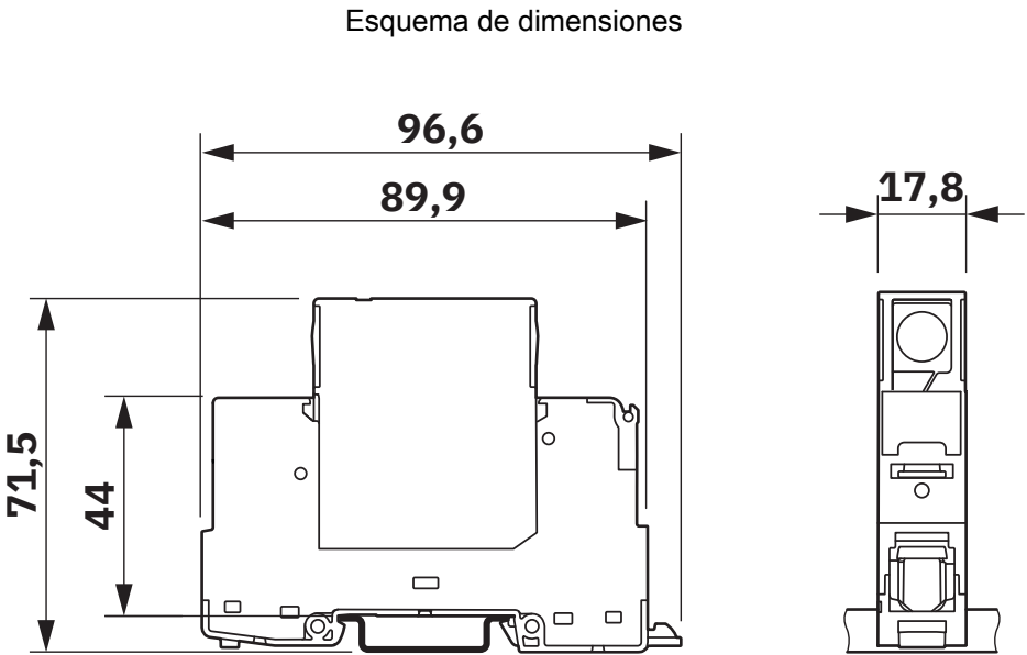
Plano esquemático
