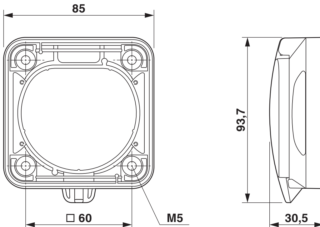
Maßzeichnung
