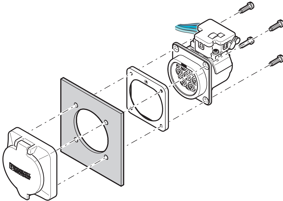
Schemazeichnung
