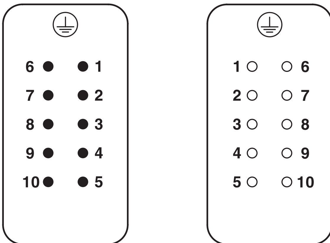
Polbild Anschlussseite
