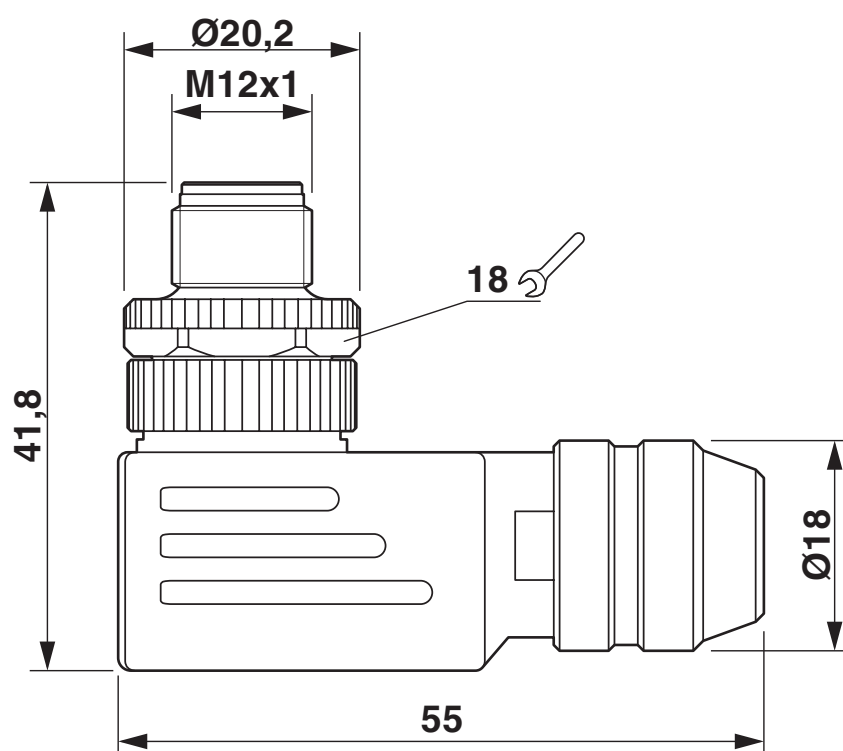
Conector macho M12 x 1, acodado, apantallado
