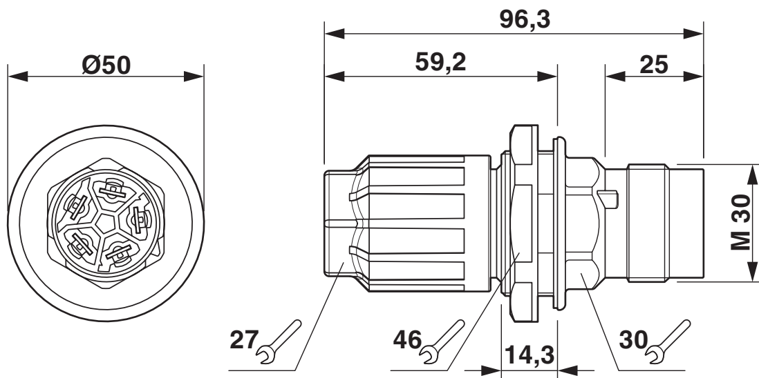
Maßzeichnung des QPD CW 5x2,5
