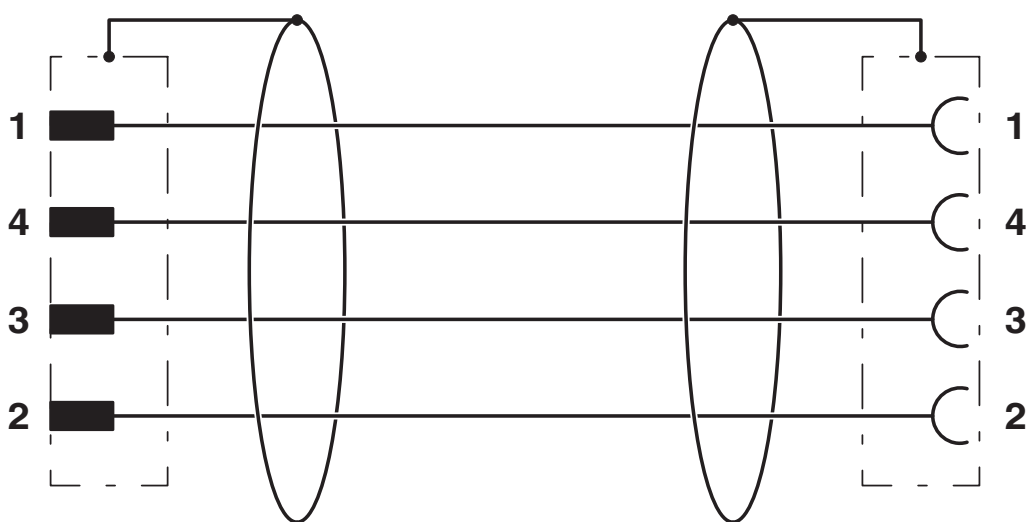
Diagrama eléctrico
