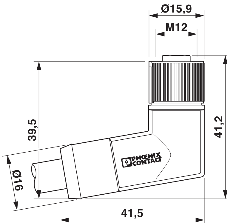
Dessin coté
