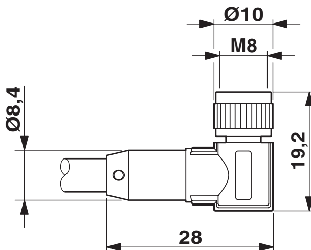
Dessin coté
