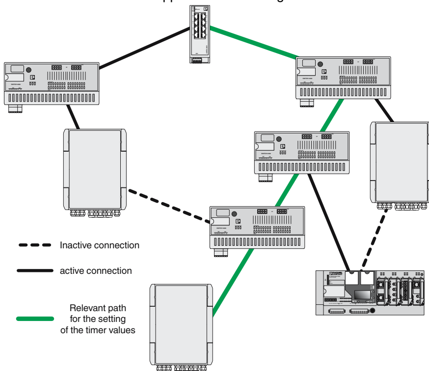
Applikationszeichnung
