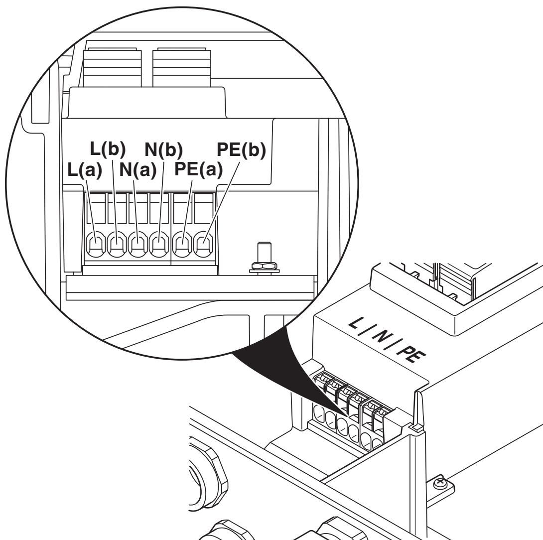
Anschlusszeichnung
