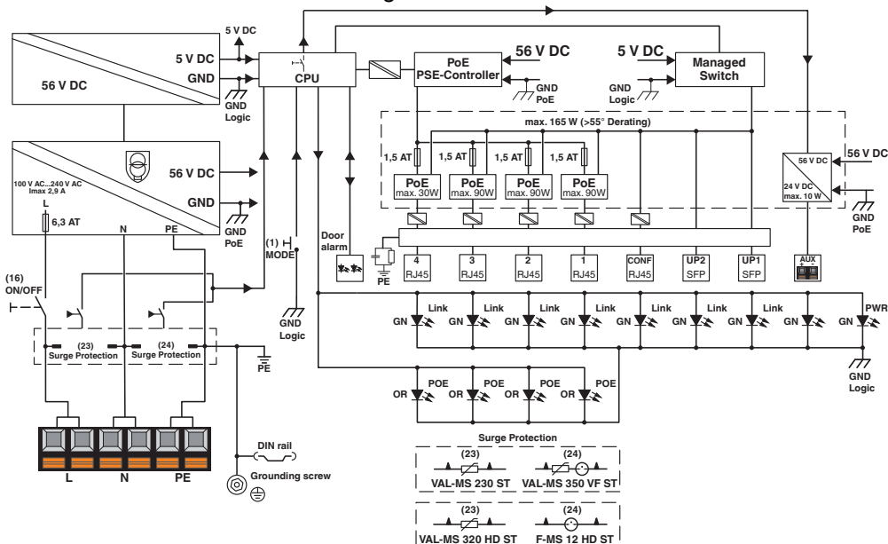
Diagrama eléctrico
