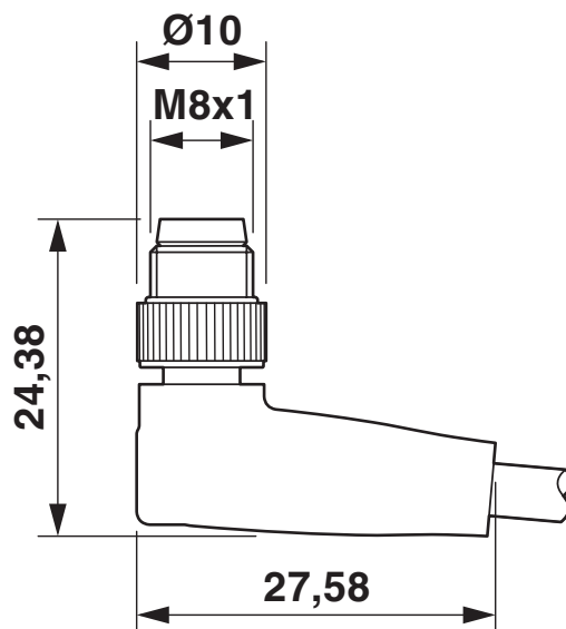
Dessin coté
