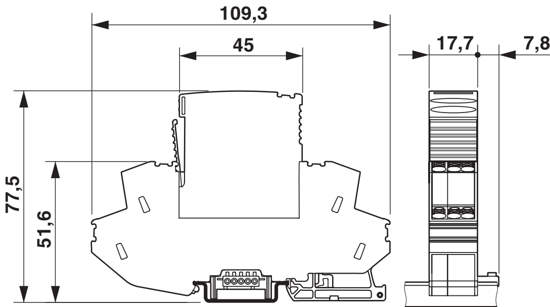
Dessin coté
